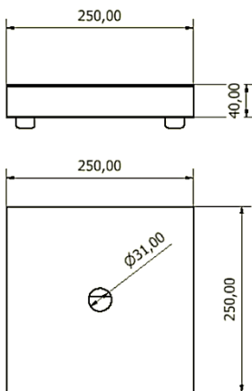
EA7-A003-2 Podstawa nablutowa
