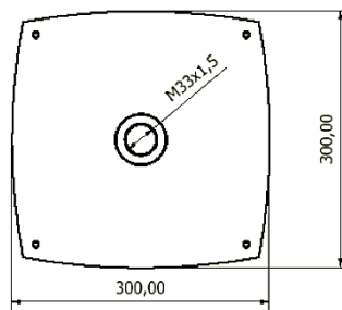
Podstawa do kolumn podłogowych (w zestawie)
