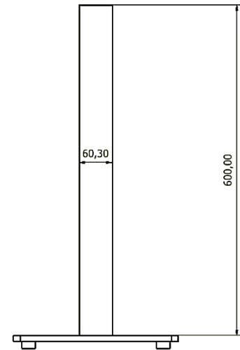
EA7-A060-2 Kolumna podłogowa 60cm
